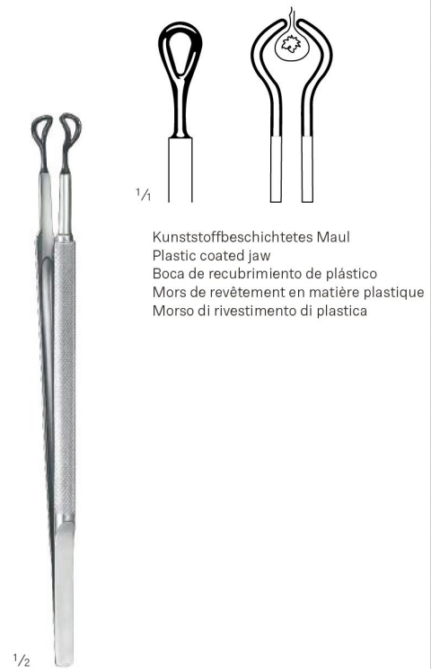
Hepp-Scheidel B03-217-18 18 cm / 7 1/8" Tubenfasspinzette Tubal forceps Pinza para tubos Pince pour saisir les trompes pinza oer afferare tubi
